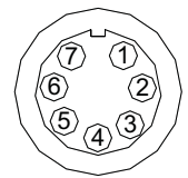
Pinout connettore Binder 712 7 pin maschio vista lato saldatura
