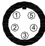
Pinout connettore Binder 712 - 5 pin femmina Vista lato terminazioni di saldatura
