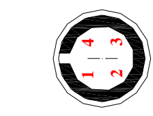
Disposition des contacts sur le connecteur Binder 719 - 4 contacts femelle Vue côté soudure
