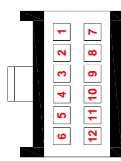
Disposition des contacts sur le connecteur AMP - 12 contacts femelle Vue côté insertion des contacts
